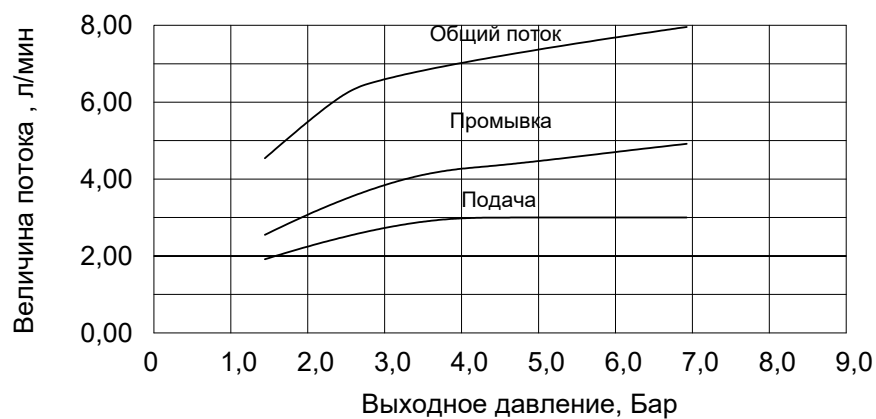
Инжектор 3 (Желтый)
