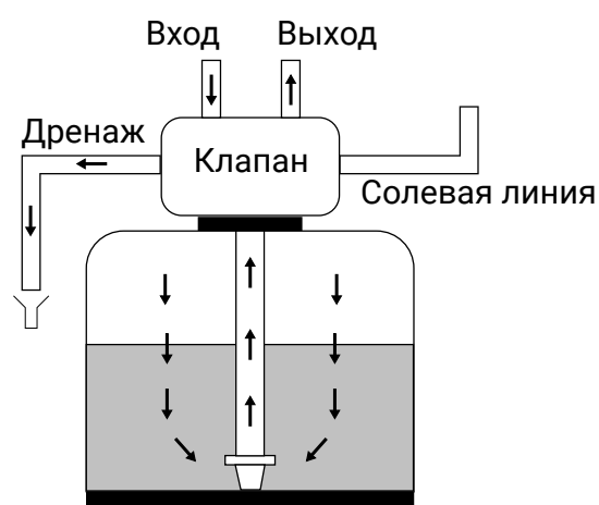
Прямая промывка
