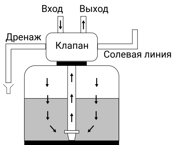
Рабочий режим
