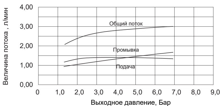
Инжектор 0 (Красный)
