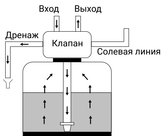
Обратная промывка
