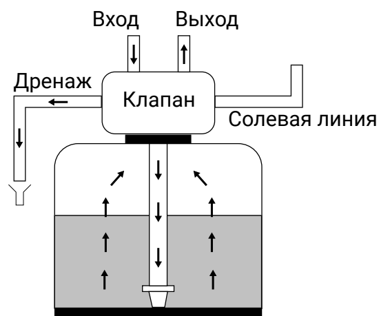
Обратная промывка
