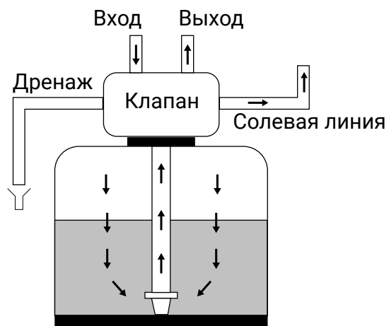
Заполнение бака-солерастворителя
