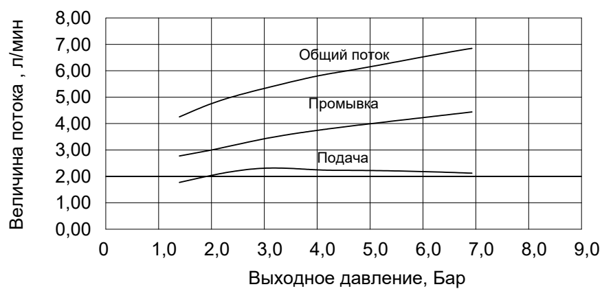
Инжектор 2 (Синий)
